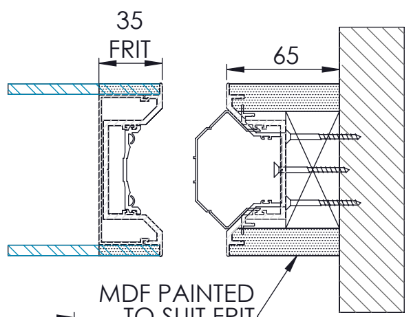
TYPE GS100 BASIC JAMB
