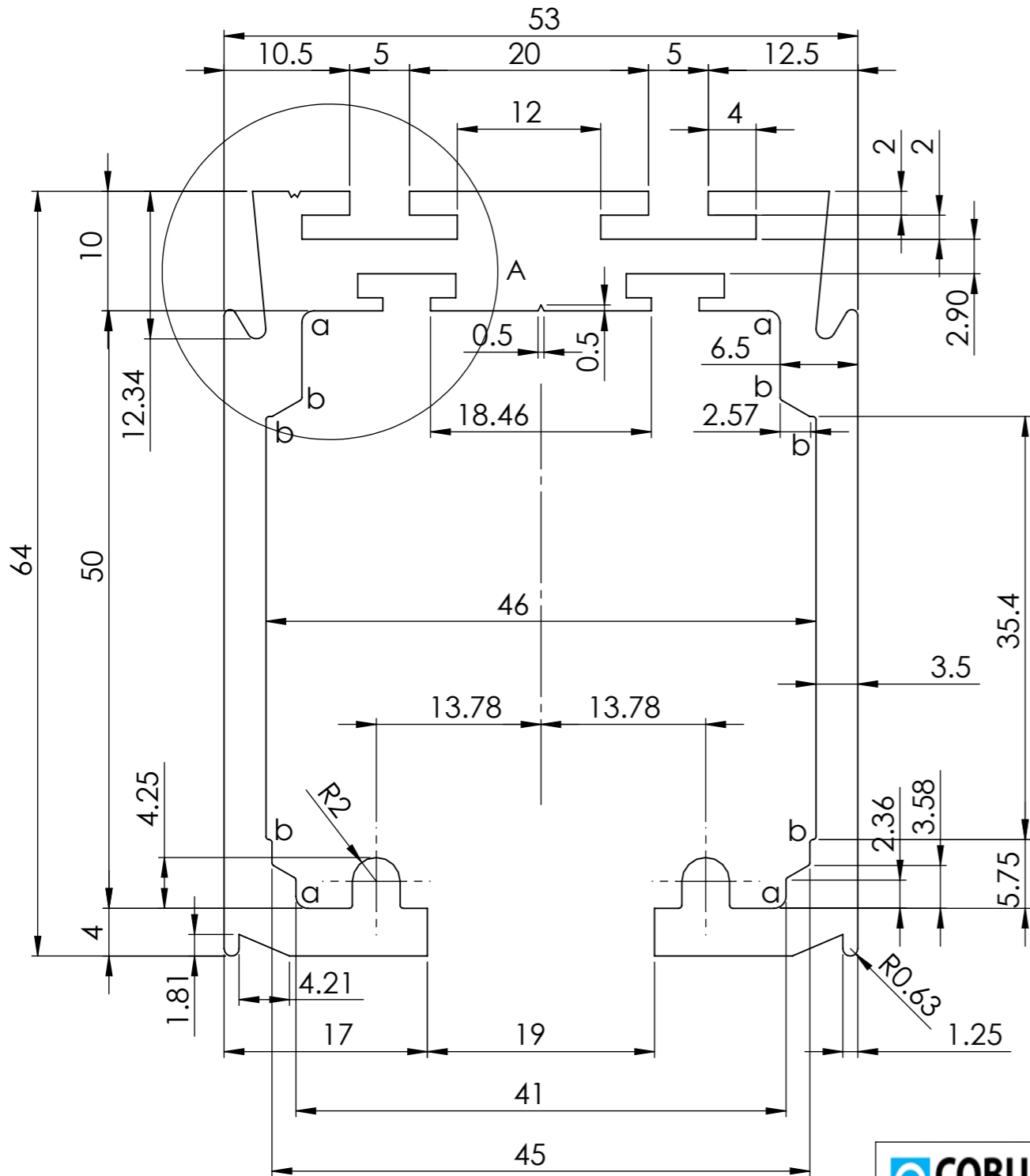
Scale 2:1
