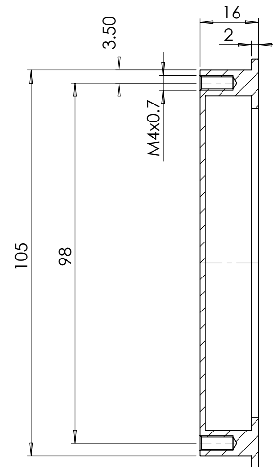
SECTION A-A
